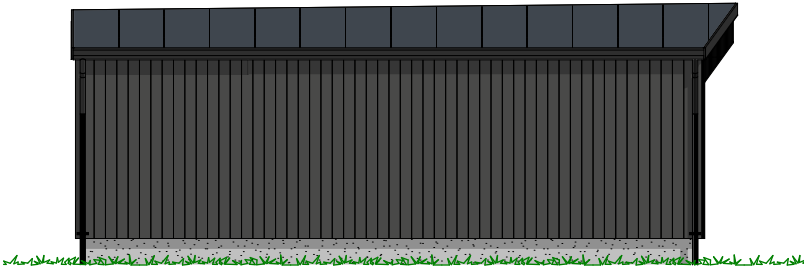
1:100 Fasade Vest
