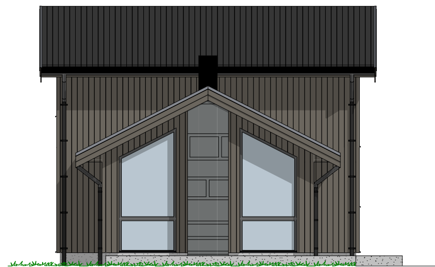
1:100 Fasade Vest
